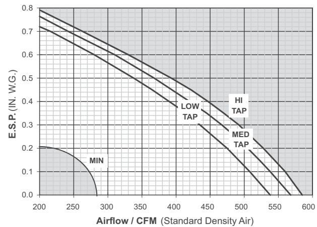
UNIT SIZE 0606
