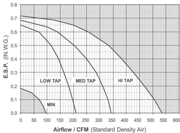
UNIT SIZES 0404, 0504, 0604, 0804
