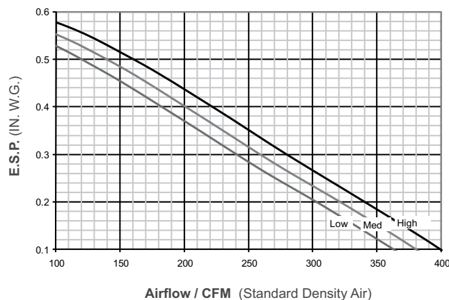
UNIT SIZE 0606, 0806, 1006
